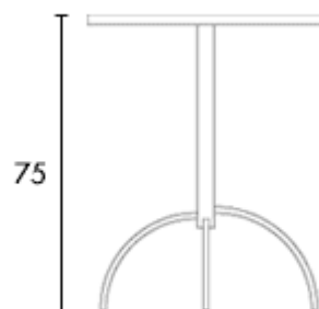
dim. Ø80 Struttura in acciaio. Piano reclinabile.
