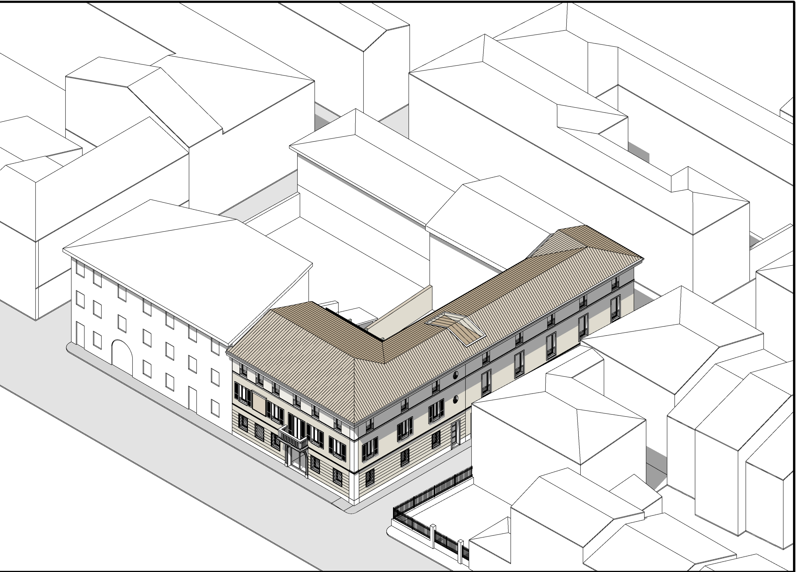
ASSONOMETRIA SUD-EST
